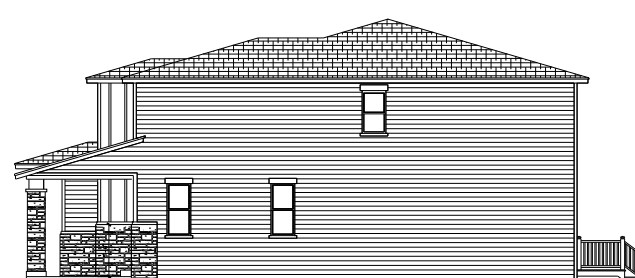
RIGHT ELEVATION
