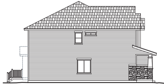
RIGHT ELEVATION
